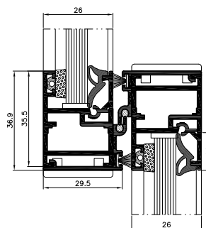
przekrój przez okno przesuwane w pionie
