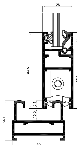
przekrój przez okno przesuwane w poziomie
